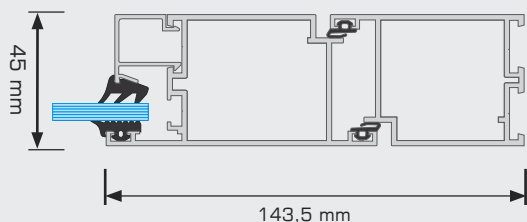
przekrój drzwi
